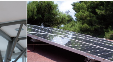
Pannelli fotovoltaici installati su tetto mediante apposita struttura di sostegno.
