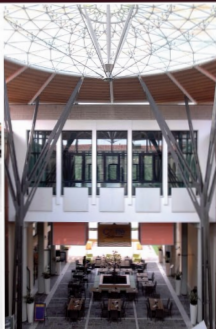
Copertura della piazzetta del Centro Culturale L. Da Vinci e del Caffè letterario - San Donà di Piave (VE)
